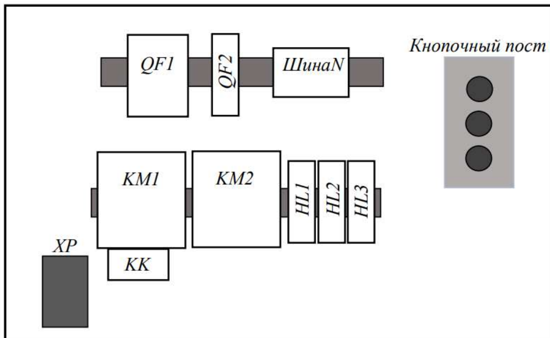
Схема компоновки реверсивного пуска асинхронного двигателя
